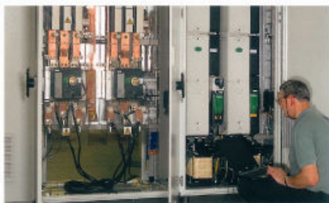
功率组件
